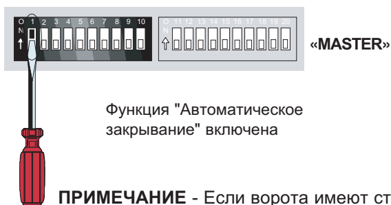
БЛОК УПРАВЛЕНИЯ "MASTER"
