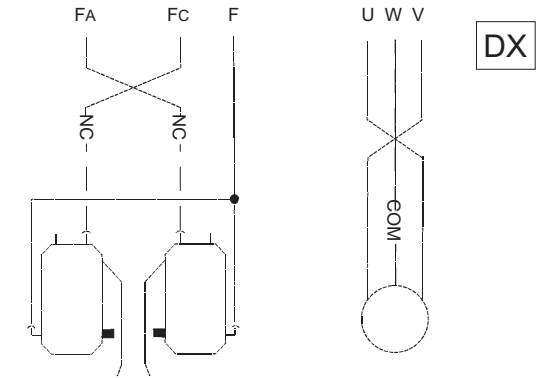
Блок микровыключателей
