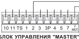
БЛОК УПРАВЛЕНИЯ "MASTER"
