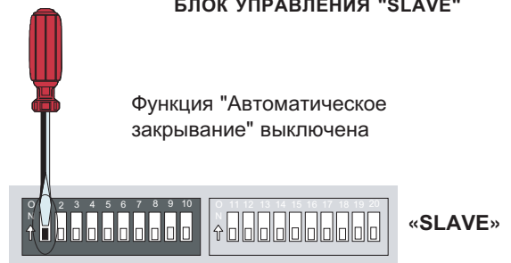
БЛОК УПРАВЛЕНИЯ "SLAVE"
